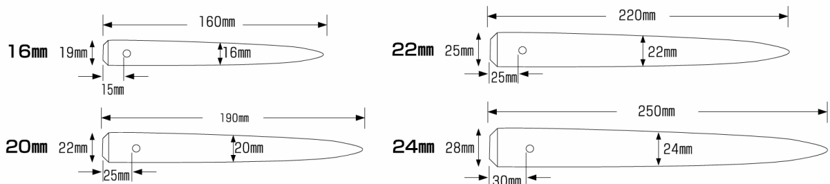
サイズ表 (穴径φ5mm)
